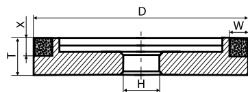
6A9 D*W*X*T*H
