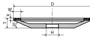
12A2-20° D*T*X*W*H
