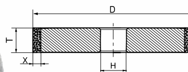
1A1 D*T*X*H
