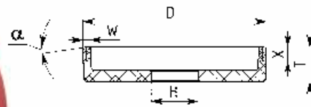
6A2 D*W*X*T*H*α°
